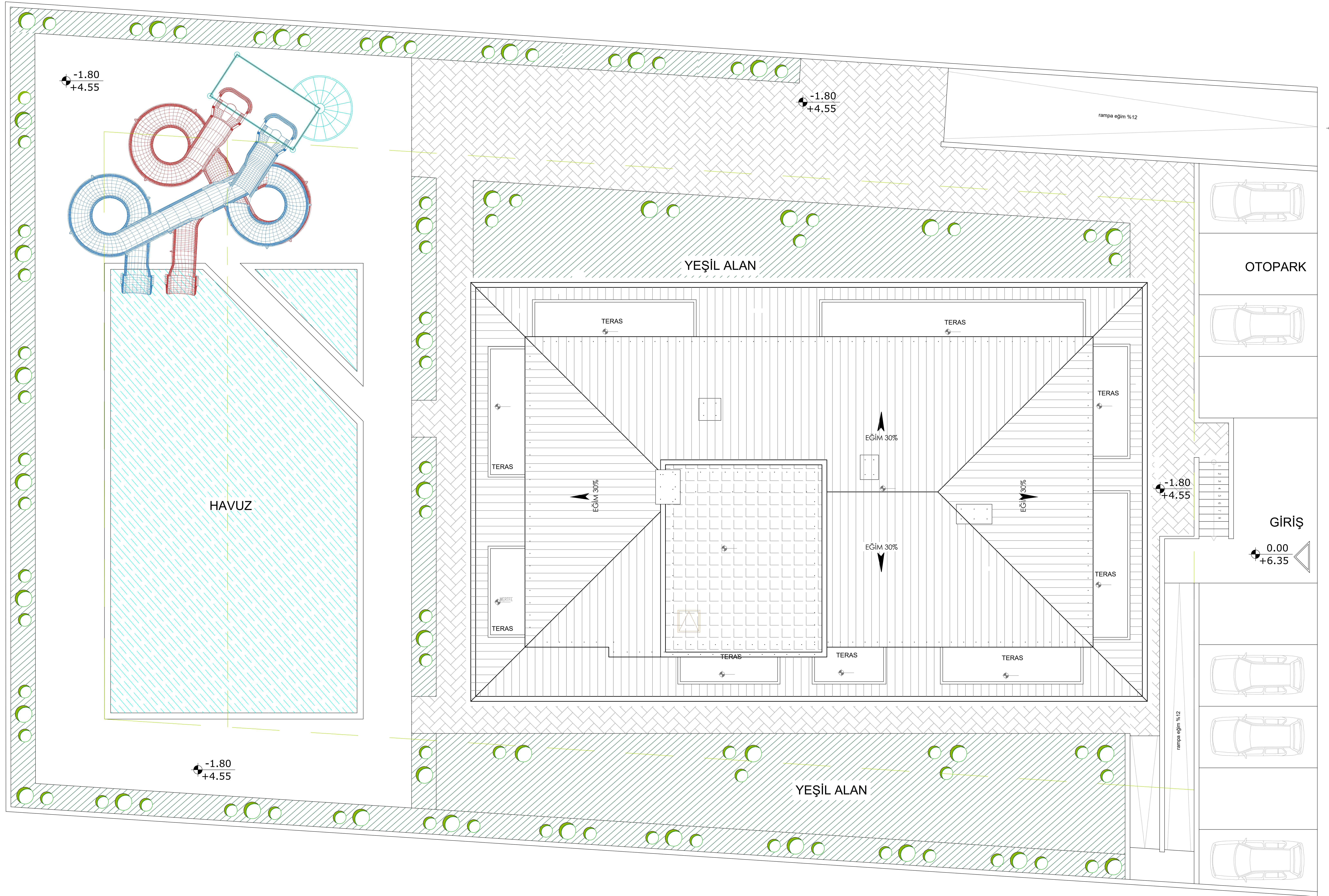
VAZİYET PLANI
