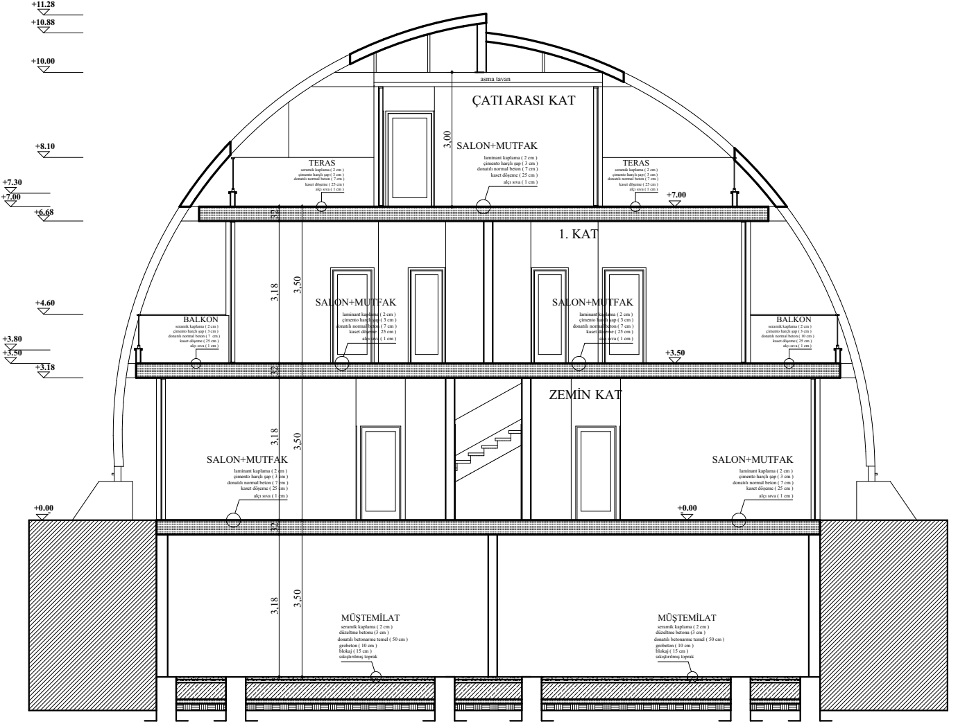
B-B KESİTİ
