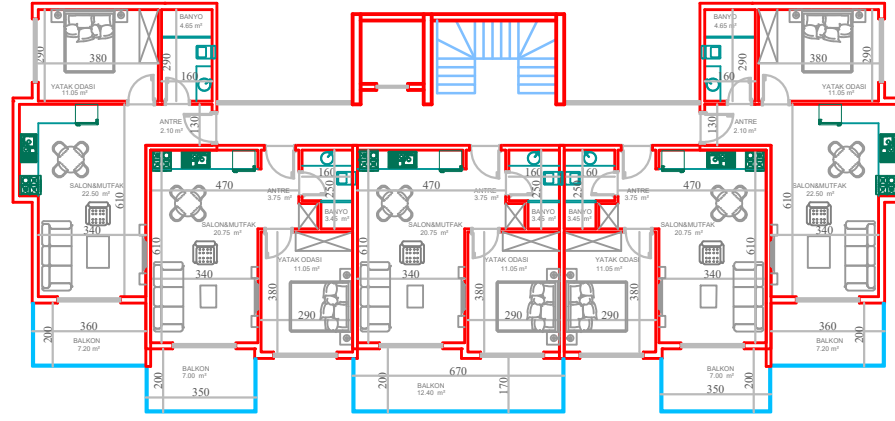
1. KAT PLANI
