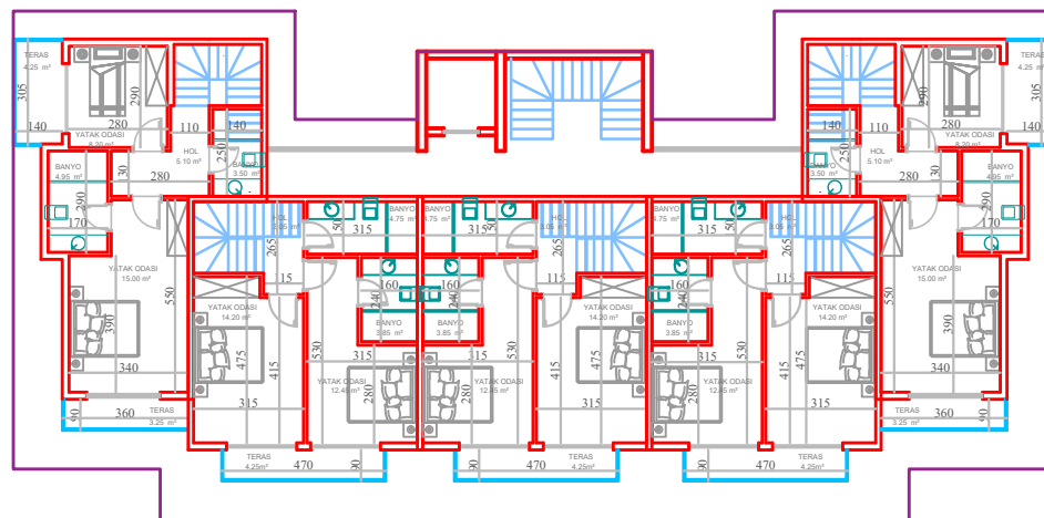
ÇATI ARASI PLANI
