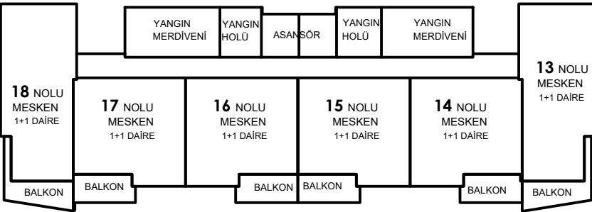
2.KAT
