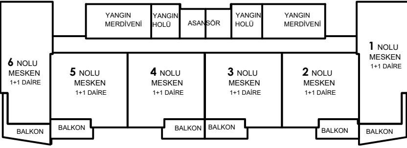
ZEMİN KAT
