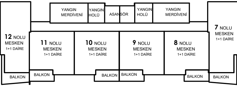
1. KAT
