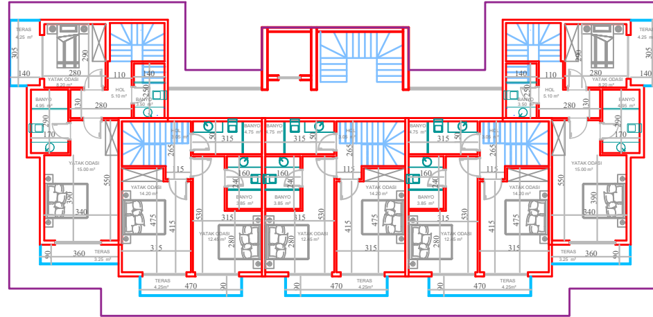
ÇATI ARASI PLANI
