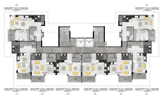
8. KAT KAT PLANI
